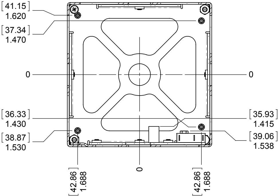
SECTION D-D
